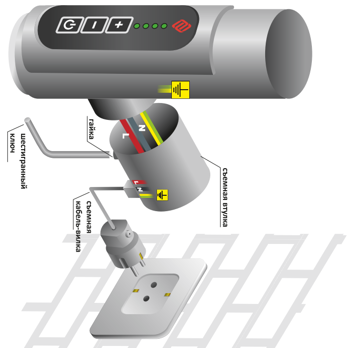
Схема 2. Подключение при помощи кабель-вилки
