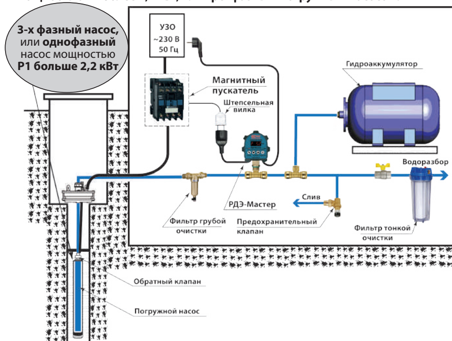
Пример 4. Подключение РДЭ-Мастер для управления однофазным насосом мощностью P1 более 2,2 кВт, или трехфазным погружным насосом.
