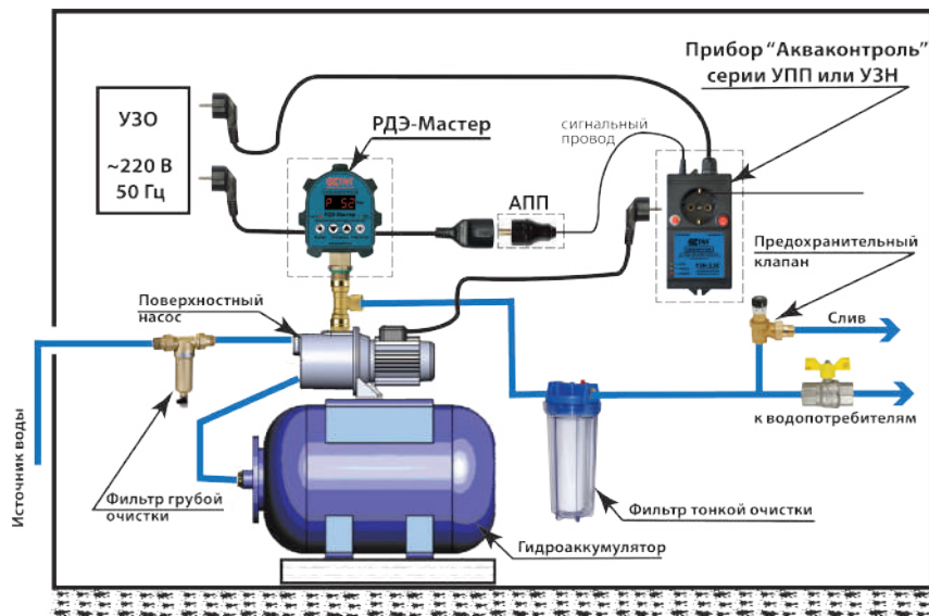
Пример 4. Подключение РДЭ-Мастер для управления однофазным насосом мощностью P1 более 2,2 кВт, или трехфазным погружным насосом.
