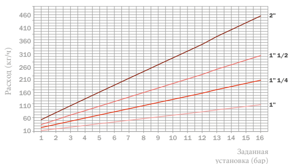
РАСХОД СПУСКА ПАРА - 1811.0-1831.0-0111.3 1"+2"
