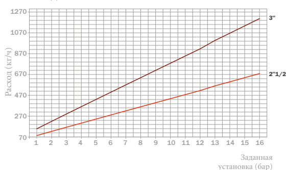
РАСХОД СПУСКА ПАРА - 1811.0-1831.0-0111.3 2"1/2+3"
