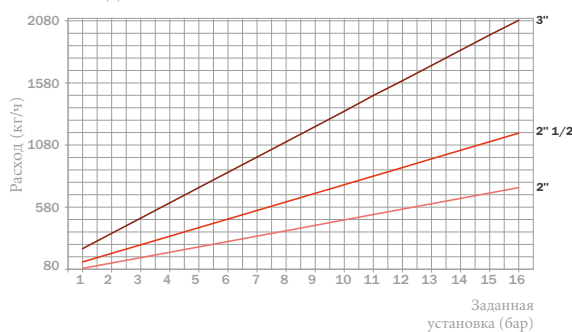
РАСХОД СПУСКА ПАРА - 1811.0-1831.0-0111.3 2"1/2+3"
