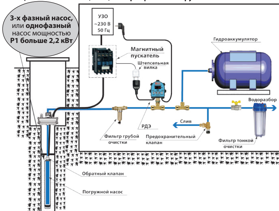
Пример 4. Подключение РДЭ для управления однофазным насосом мощностью P1 более 2,2 кВт, или трехфазным погружным насосом.
