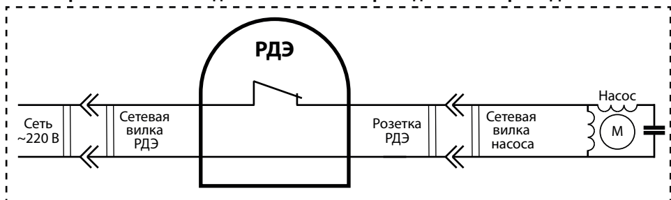
Электрическая схема подключения насоса к реле давления серий БРД
