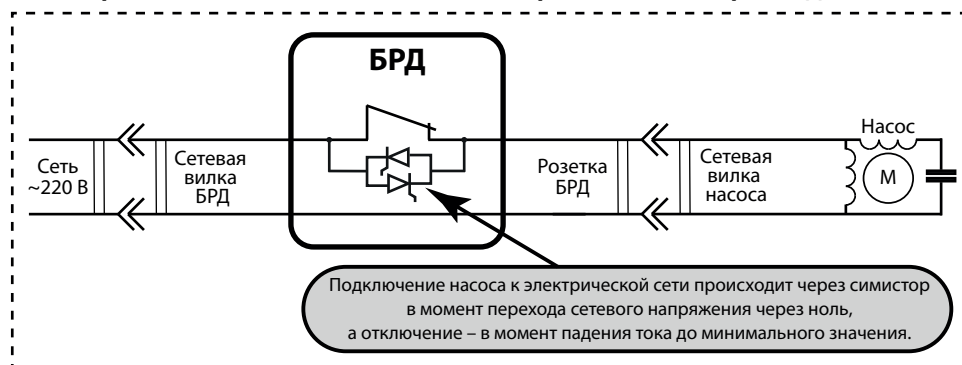
Электрическая схема подключения насоса к реле давления серий БРД
