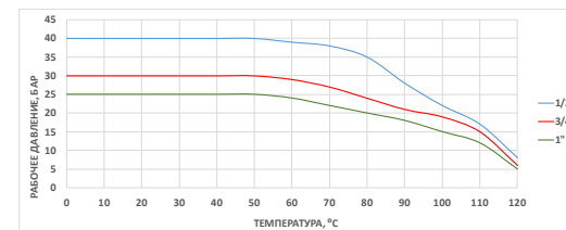
График зависимости рабочего давления от температуры
