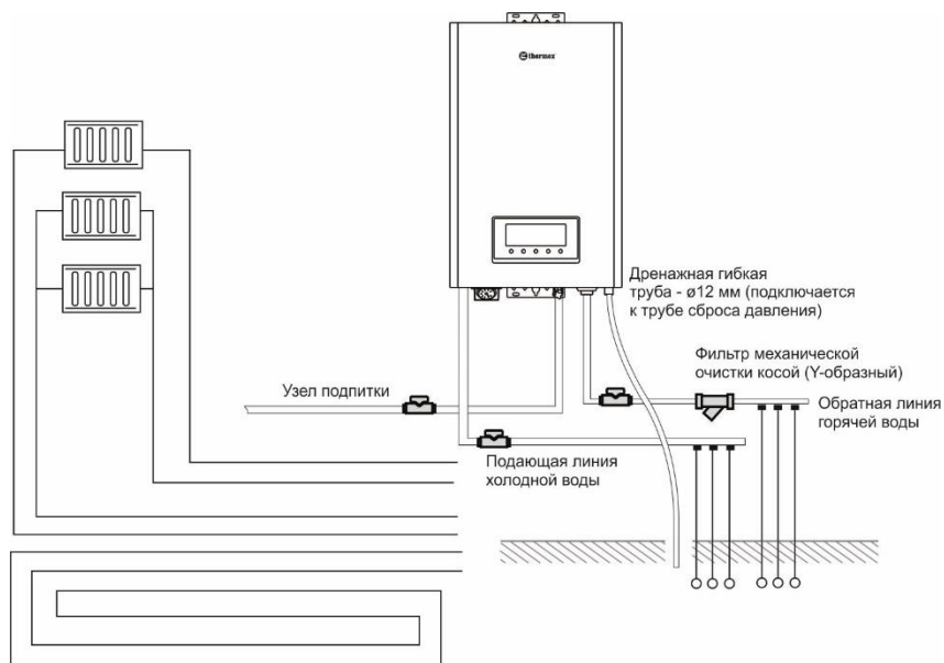
Рис. 4. Схема подключения труб
