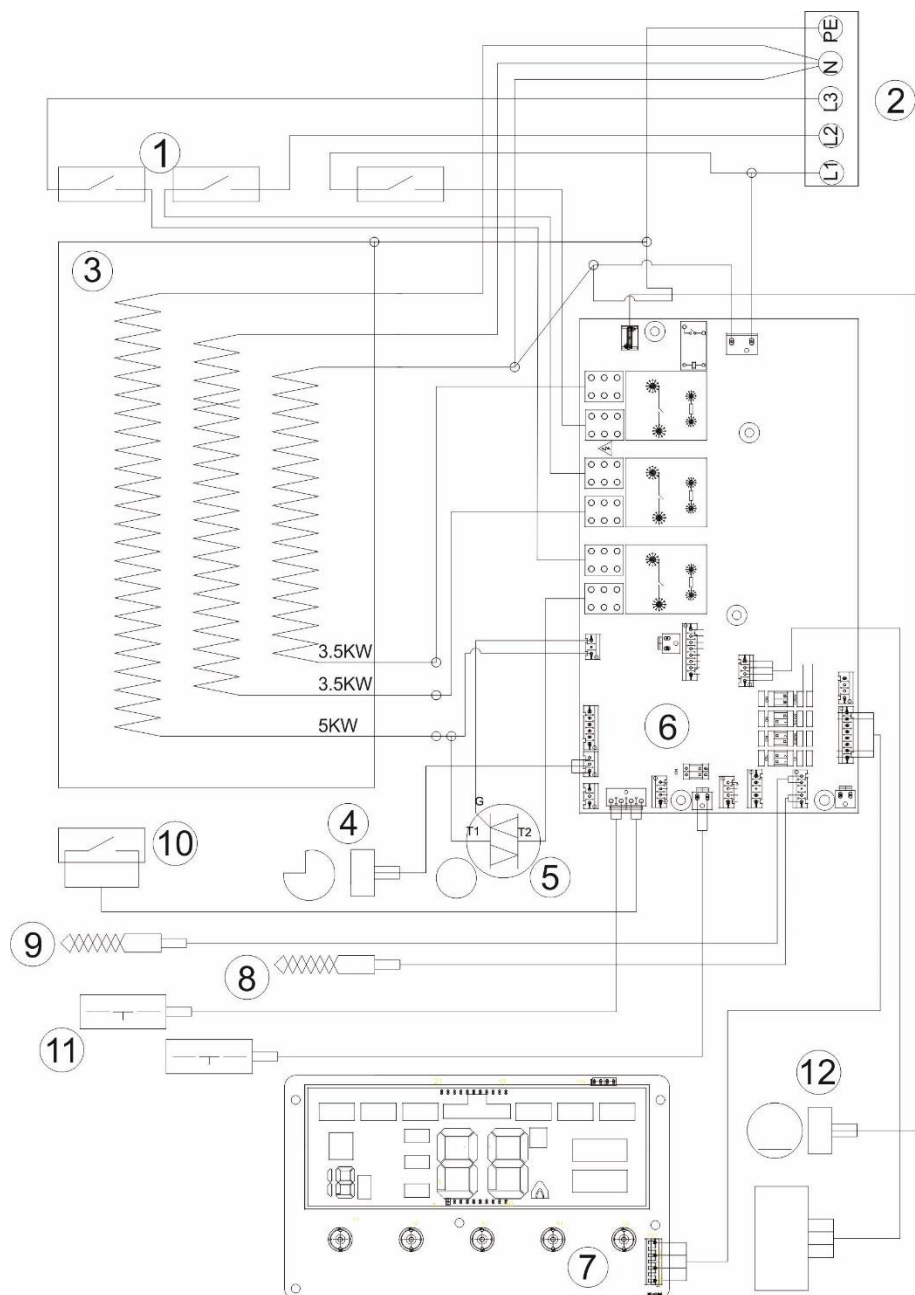
Рис. 15. Электрическая схема THERMEX Grizzly 5-12 Wi-Fi
