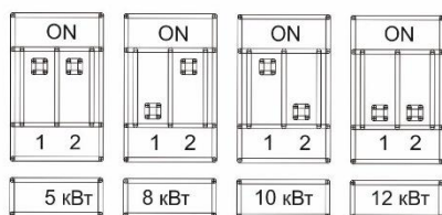
Рис. 9. Положение рычагов переключателя мощности.
